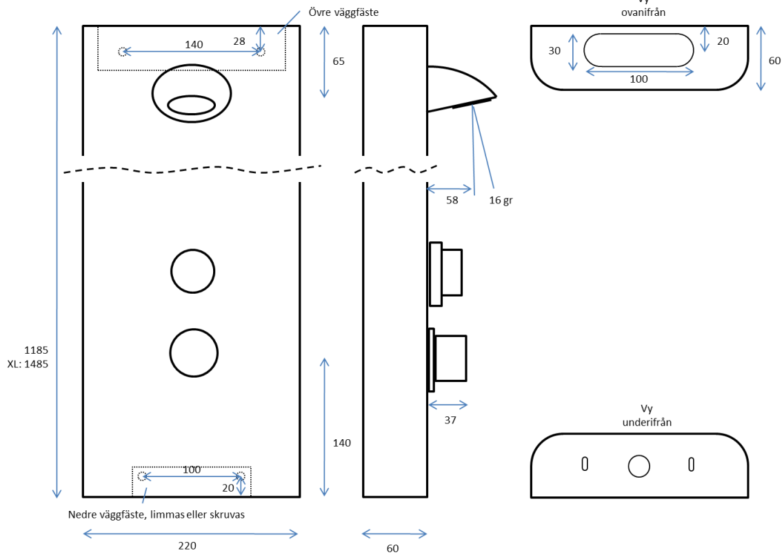
Måttskiss ACSS Duschpanel 101, 131
