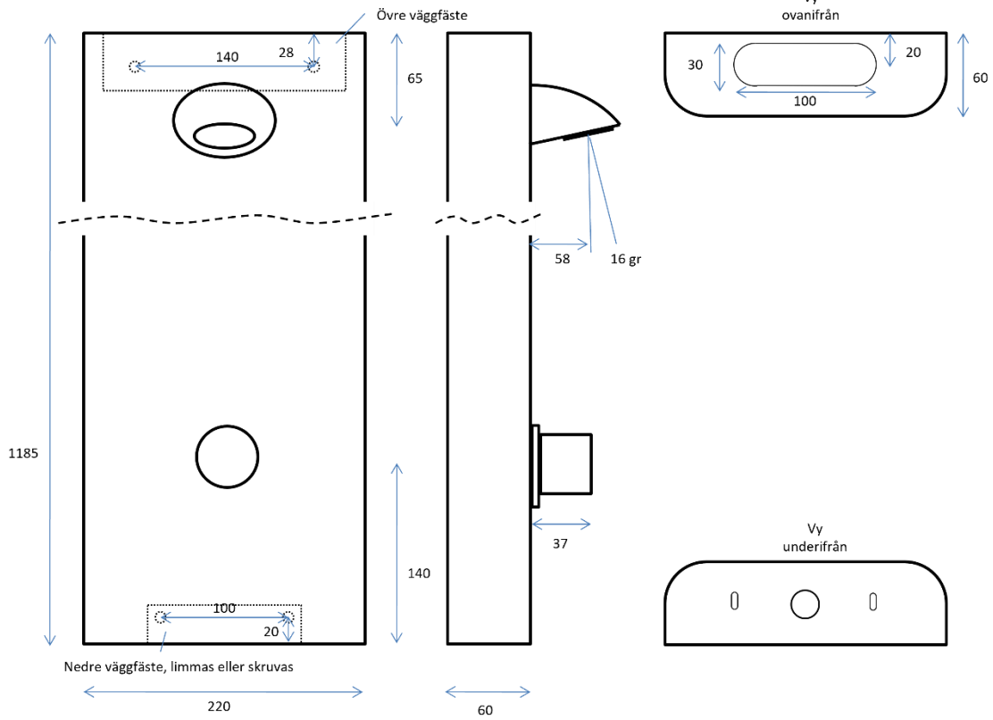
Måttskiss ACSS Duschpanel 100, 130
