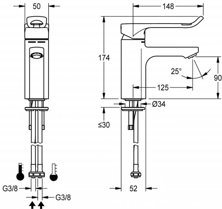
Måttskiss 24215.202.300:
