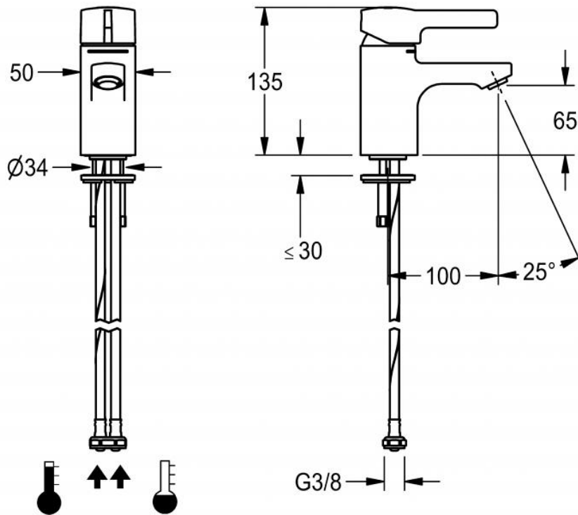
Måttskiss 24215.202.300:
