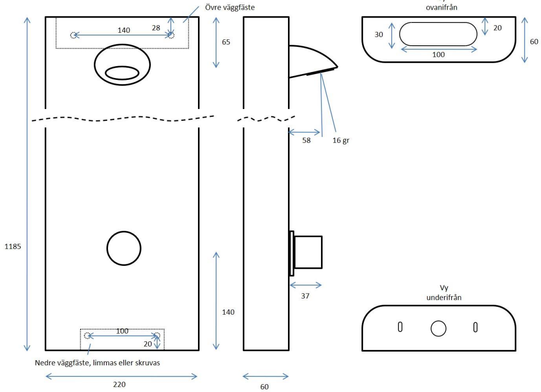
Måttskiss ACSS Duschpanel 130
