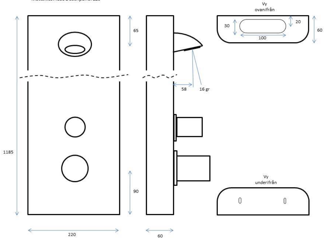
Måttskiss ACSS Duschpanel 120
