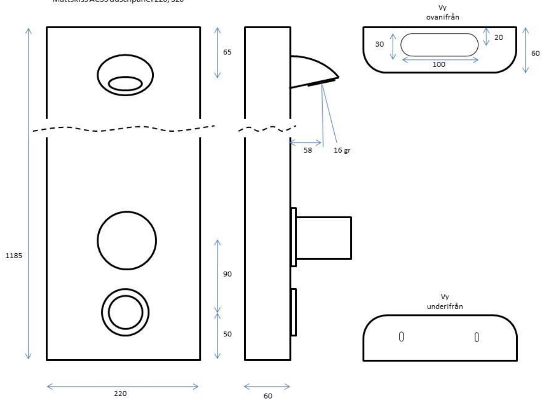
Måttskiss ACSS duschpanel 220, 320
